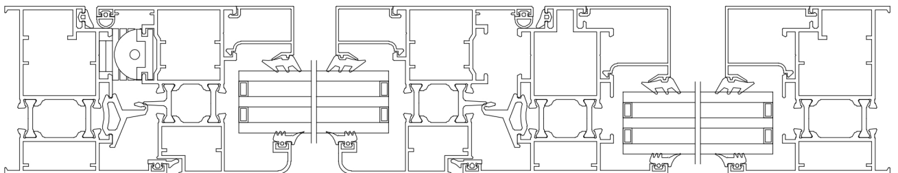
A-A
