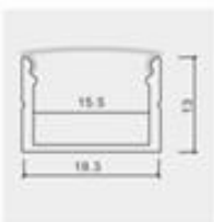
Model: ZJD-LS2013 Size:Lx19.3x13mm PCB:15mm
